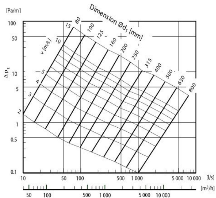
Tlaková ztráta
