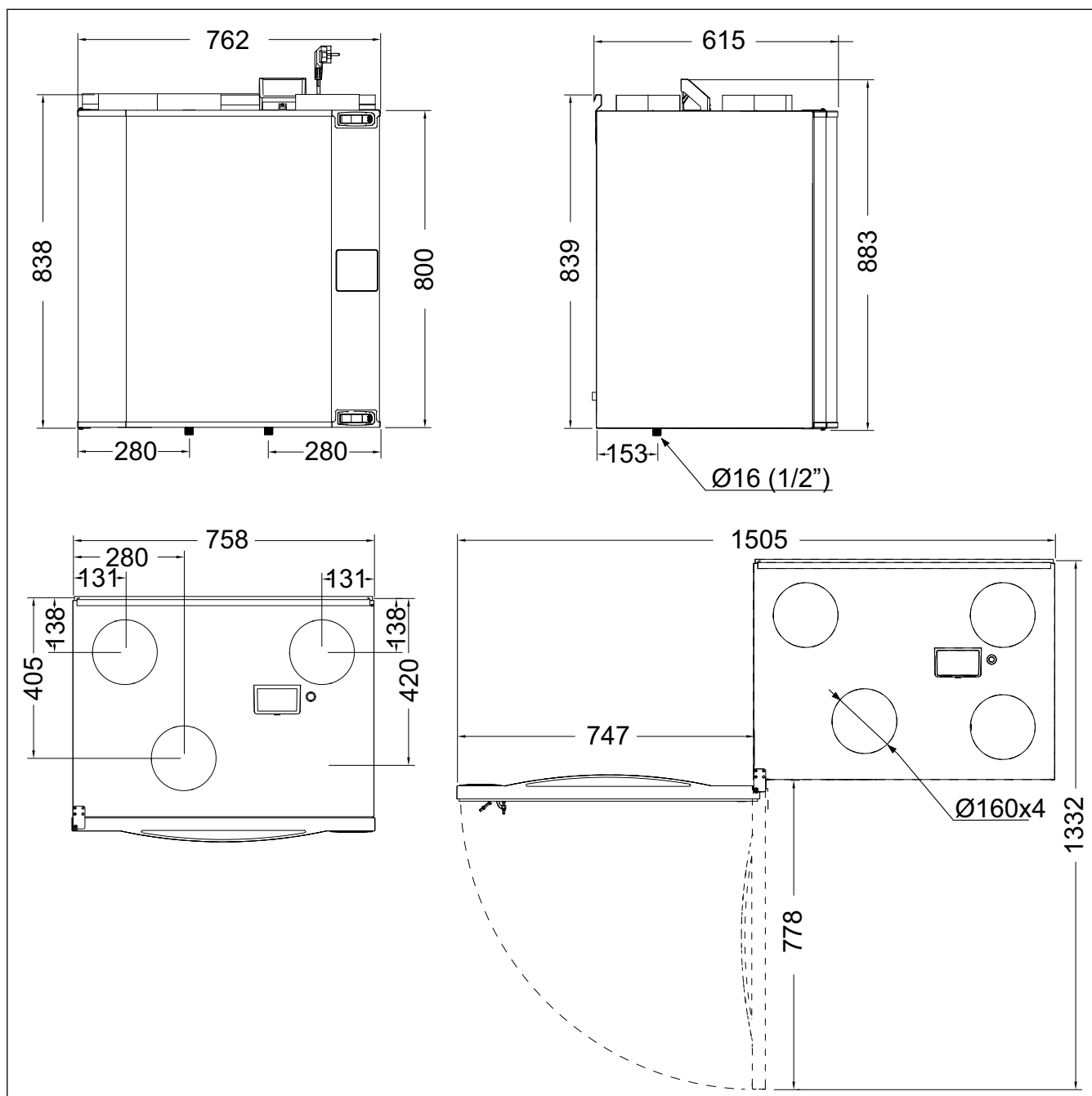
Obr. 2 Pravý model (přívod čerstvého vzduchu je umístěn na pravé straně)
