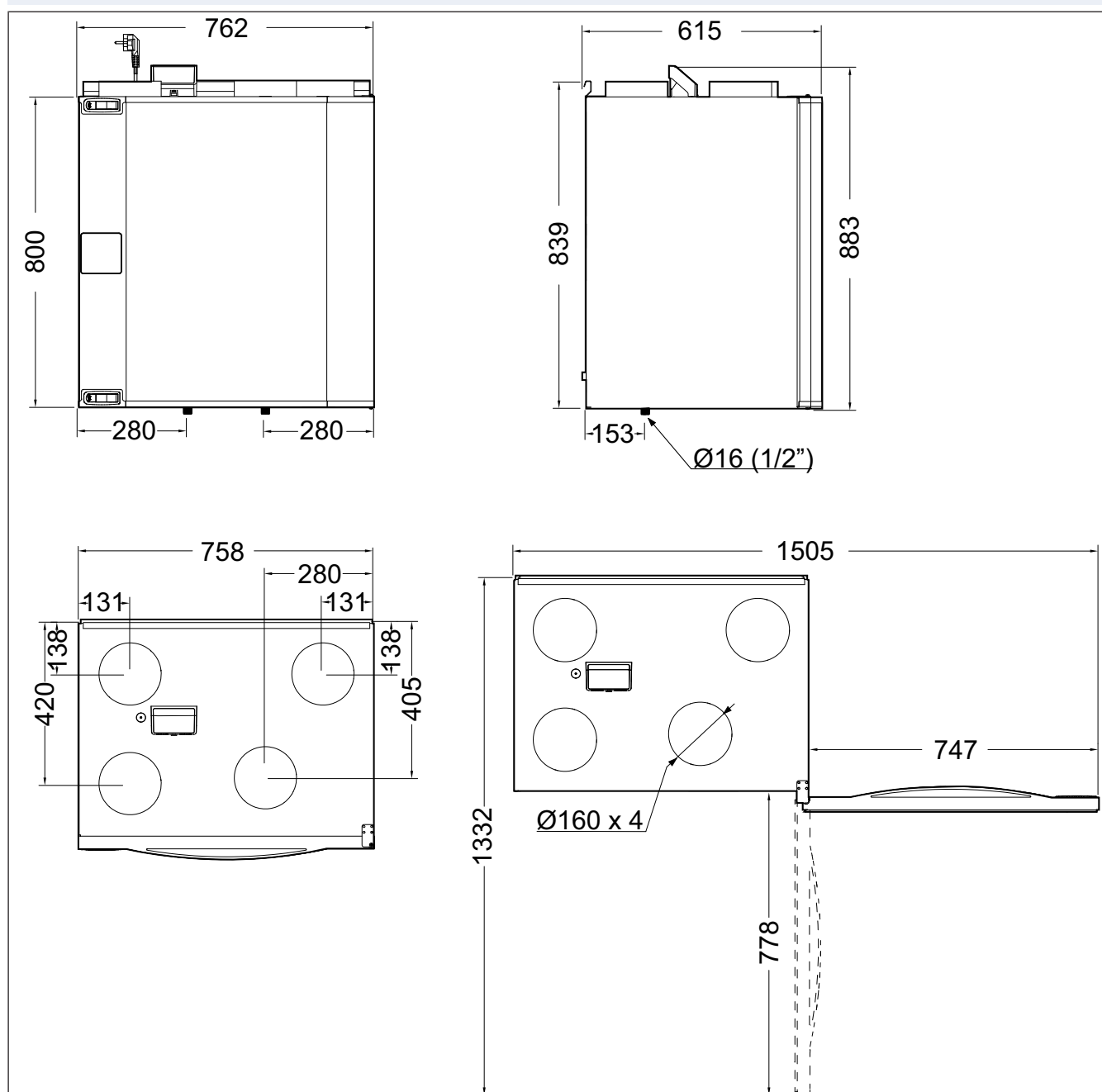
Obr. 1 Levý model (přívod čerstvého vzduchu je umístěn na levé straně)
