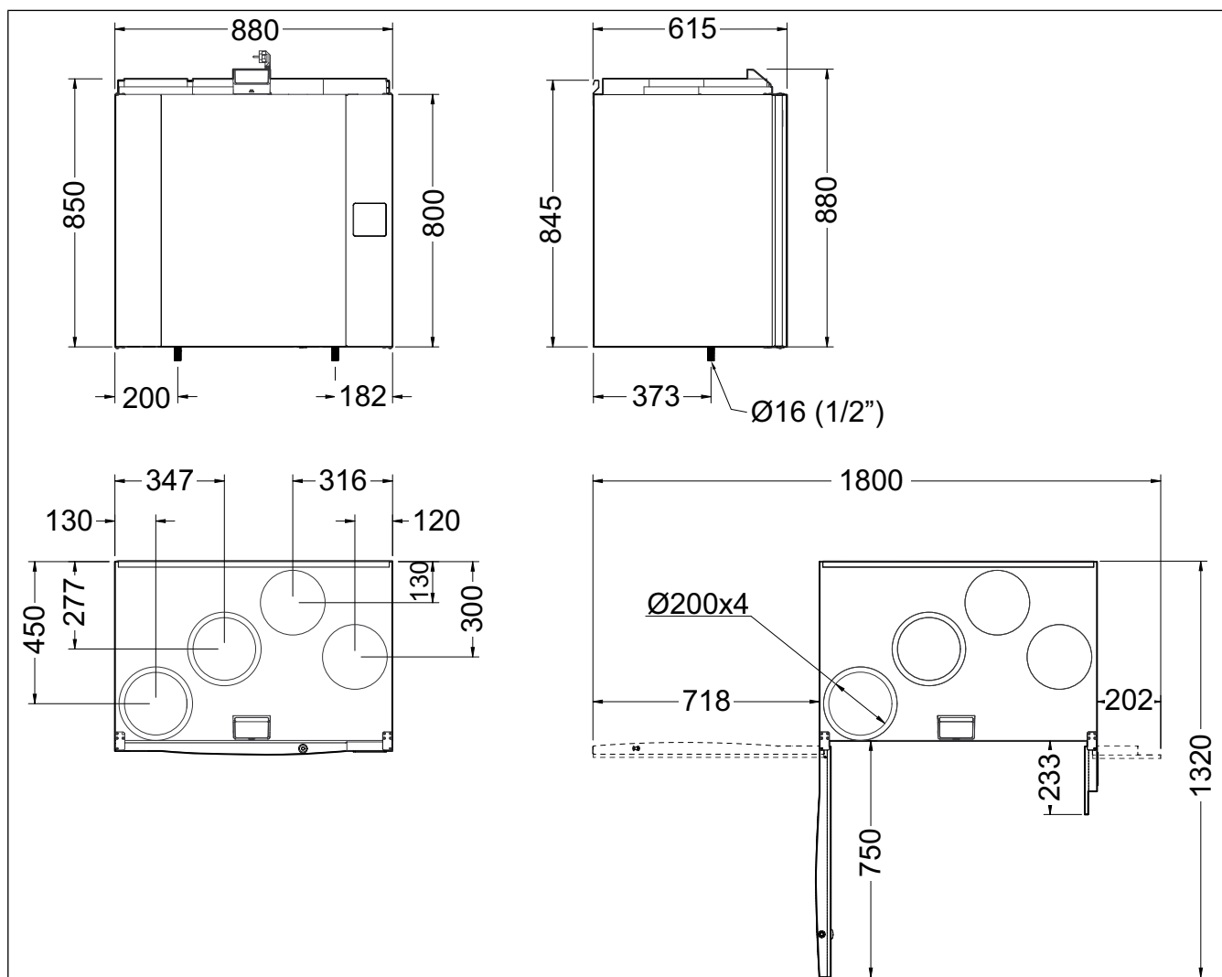
Obr. 2 Pravý model (přívod čerstvého vzduchu je umístěn na pravé straně)
